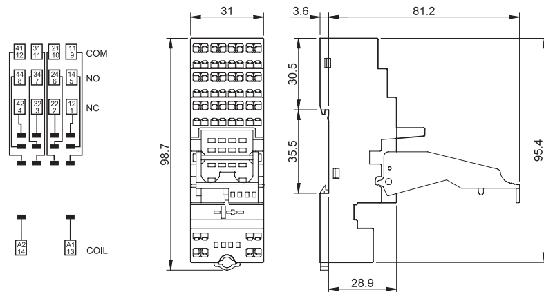
Fassung + Kammbrücke
