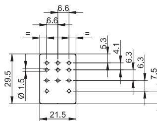
Ansicht auf die Anschlüsse
